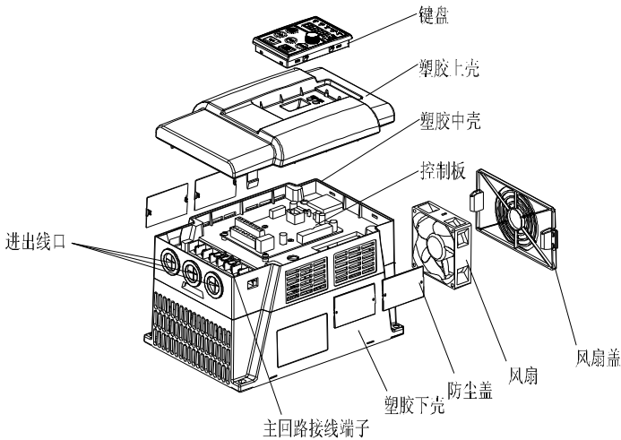
图 2-4 5.5kW-7.5kW 组件图
