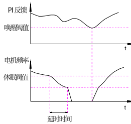
图 5-7-2 休眠和唤醒
