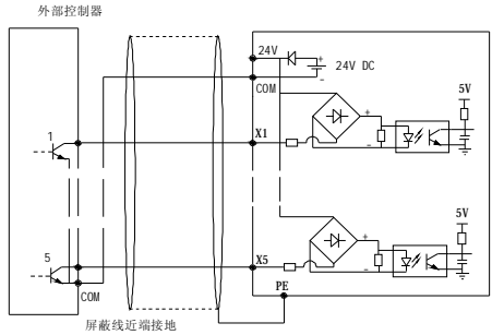
图2-22输入多功能端子配线连接图
