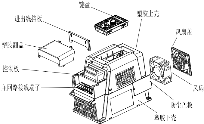
图 2-3 4kW 及 4kW 以下组件图
