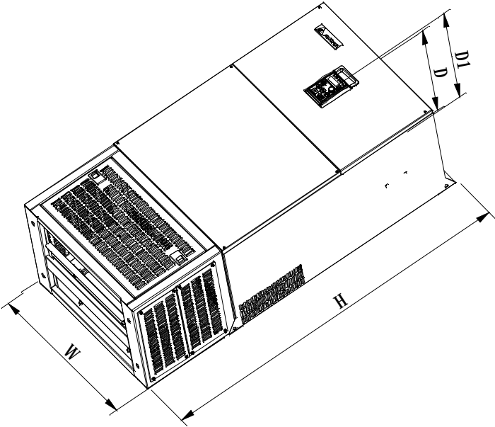
外形尺寸 (单位: mm)
