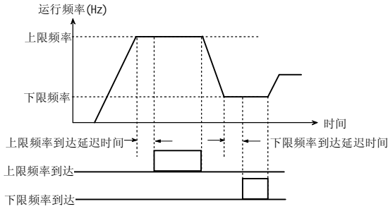
图 5-3-10 上下限频率到达
