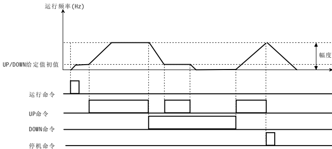
图 5-3-4 UP/DN 端子非组合运行
