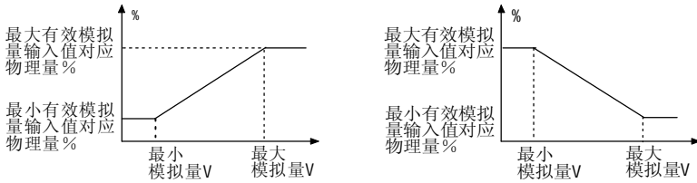
图 5-4-1 模拟输入线性曲线
