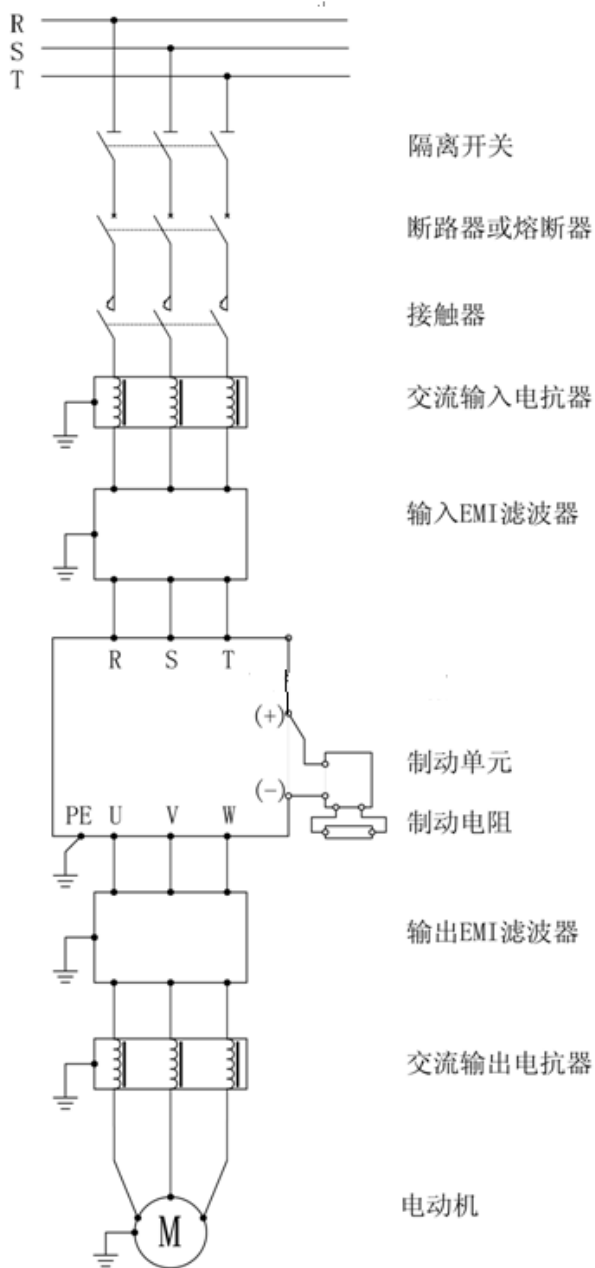
图 7-2 3018G/3022P 及以上外围设备连接图
