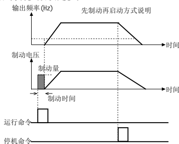
图 5-1-1 启动制动
