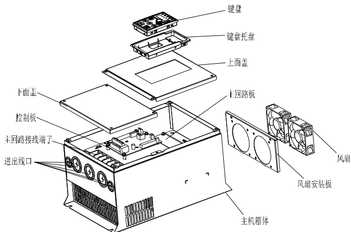
图 2-5 11kW-160kW 组件图
