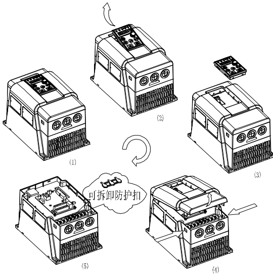
图 2-7 5.5kW-7.5kW 以下拆装示意图
