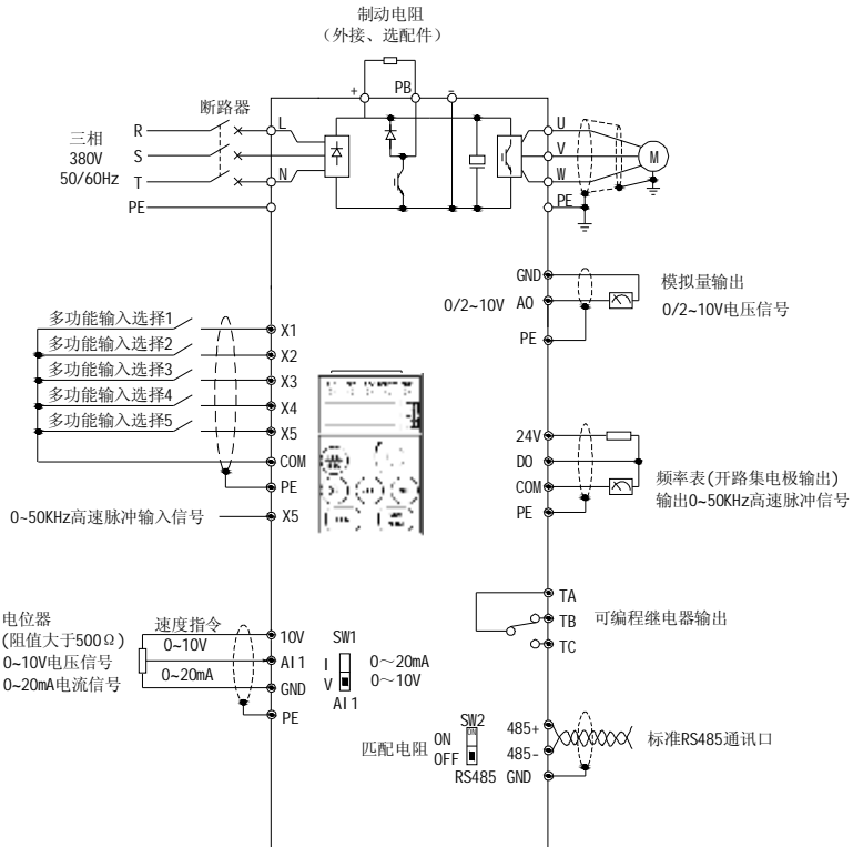
图 2-25 接线图
