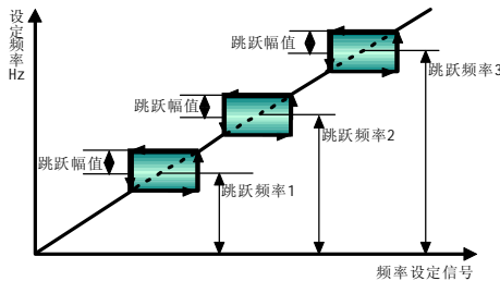
图 5-2-5 跳跃频率
