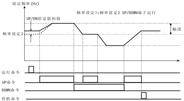
图 5-3-3 UP/DN 端子组合运行
