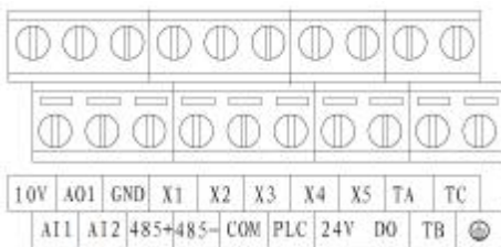
图 2-15 S2R4GB~S2R75GB 控制回路端子排布
