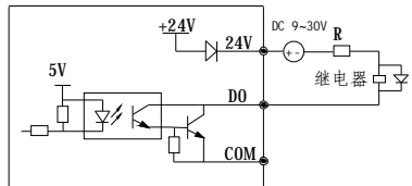
图 2-24 多功能输出端子开关量输出接线方式2
