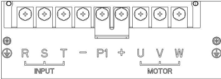
图 2-13 3PH 380V 37-160kW 主回路端子接线
