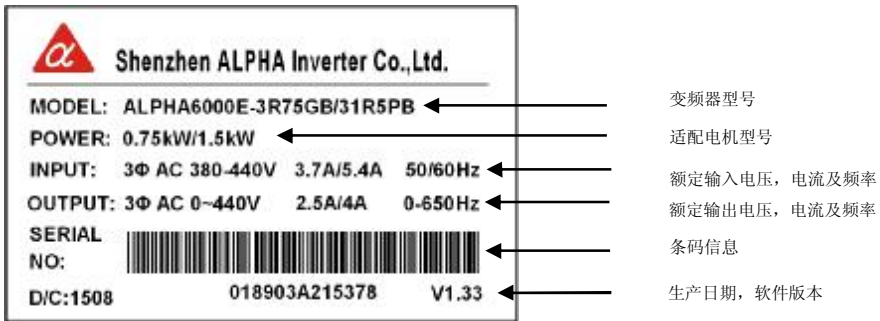
图 1-2 铭牌说明
