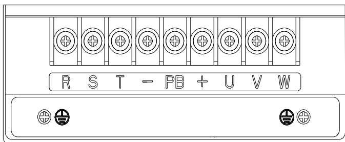
图 2-11 3PH 380V 4-15kW 主回路端子接线
