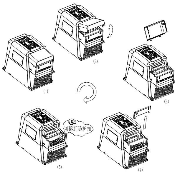
图 2-6 4kW 及 4kW 以下拆装示意图
