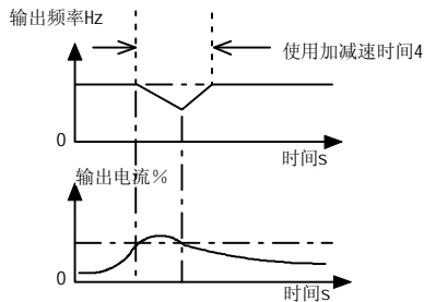
图 5-13-4 稳定运行过程
