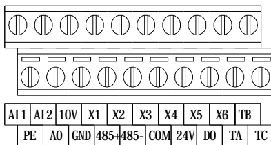
图 2-16 S21R5GB~S22R2GB, 3R75GB/31R5PB 及以上功率产品控制回路端子排布
