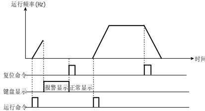
图 5-3-1 端子复位
