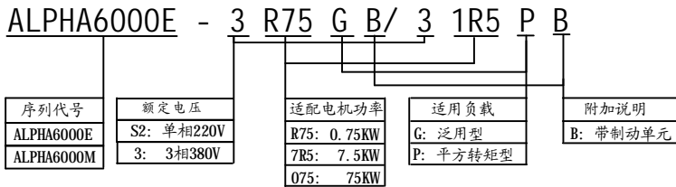
图 1-1 型号说明
