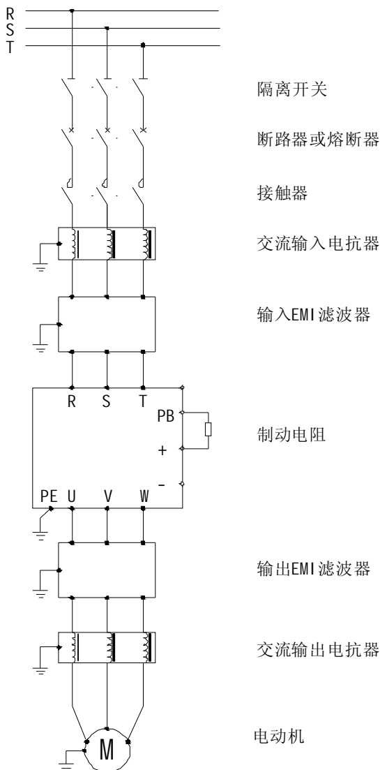
图 7-1 S2R4GB-3015GB/3018PB 外围设备连接图
